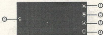
Android kód
